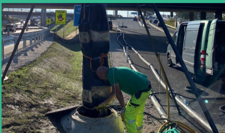
Einbau Rohrdichtkissen
