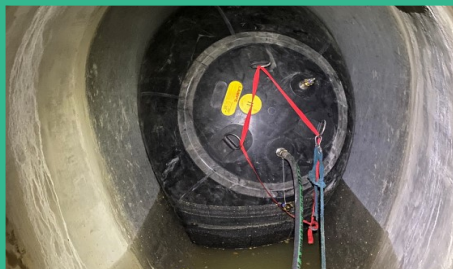
Eingebautes Rohrdichtkissen
